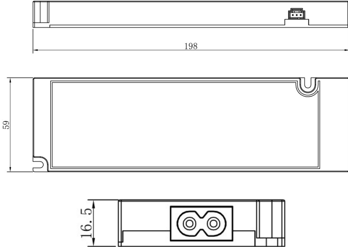
13-1 外形图 单位: mm
