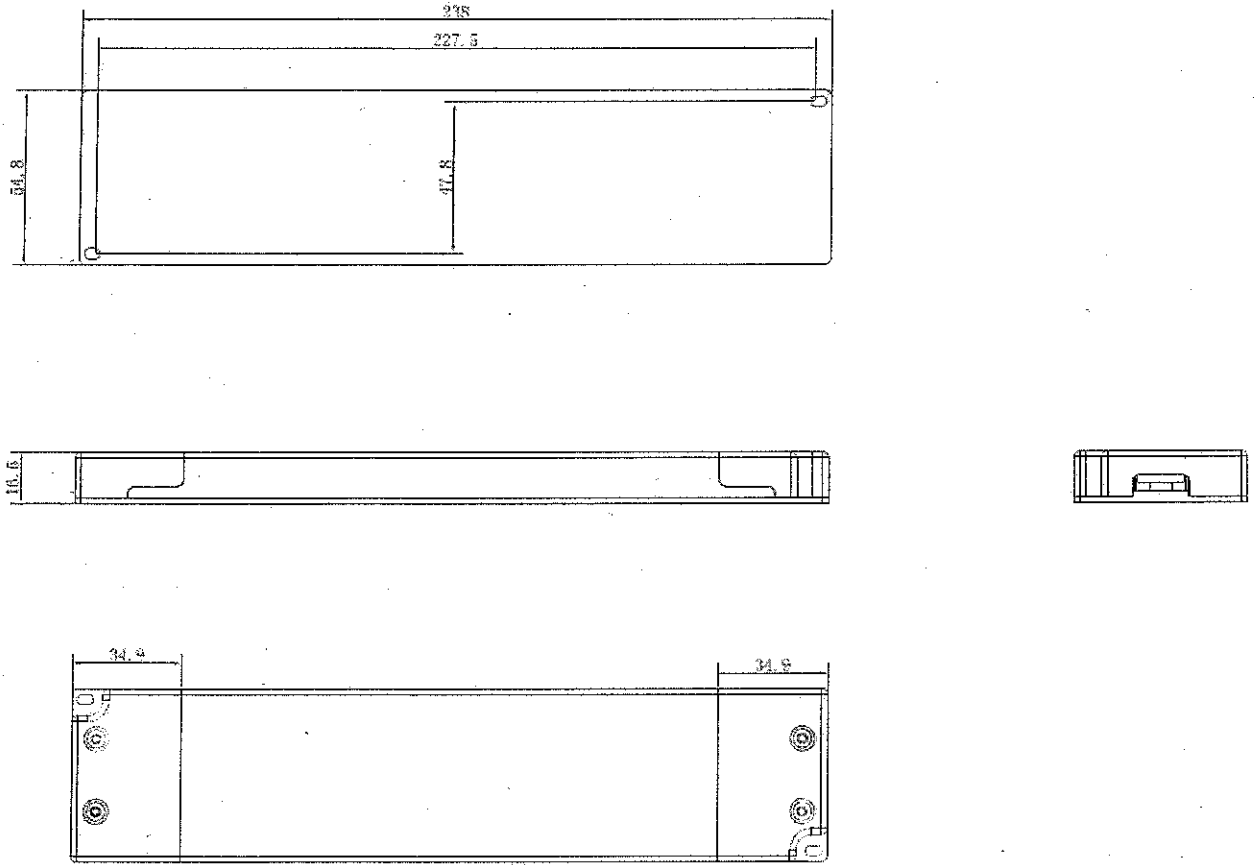
12-1 外形尺寸 单位 (mm)
