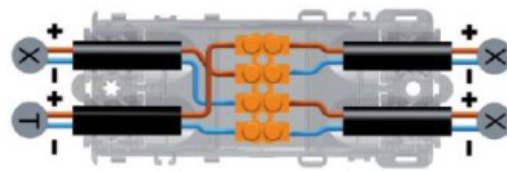
Schema 1: Collegamento in serie di 3 faretti LED con alimentatore
