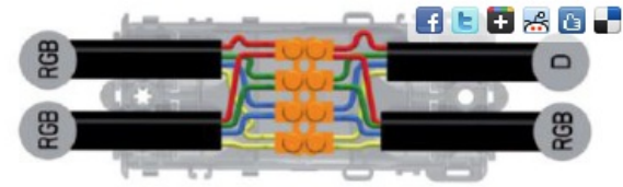
Schema 2: Collegamento in parallelo di 3 faretti LED RGB (cavo con 4 conduttori) al driver RGB
